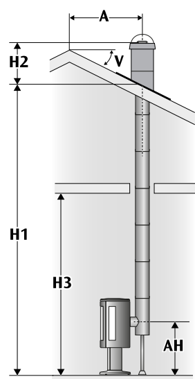
2B - Bakansluten direkt bakom eldstad. Helisolerad skorsten.
