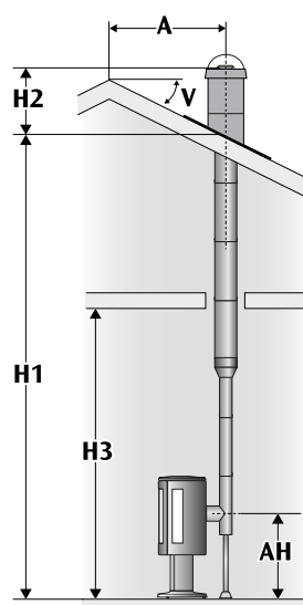
3B - Bakansluten direkt bakom eldstad. Oisolerat startör.
