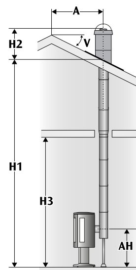
1B - Bakansluten direkt bakom eldstad. Halvisolerat startör med övergång dold i bjälklag
