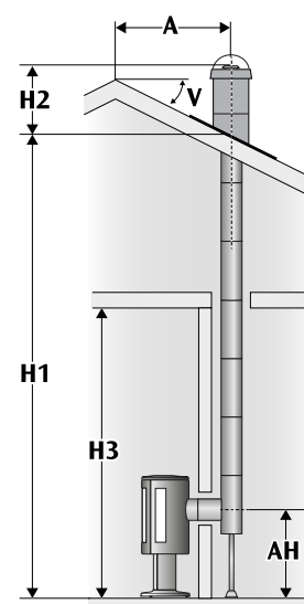
1BM - Bakansluten genom mellanvägg
