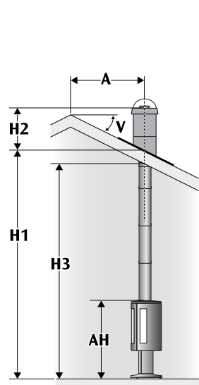
T - Toppmonterad - halvisolerad.
