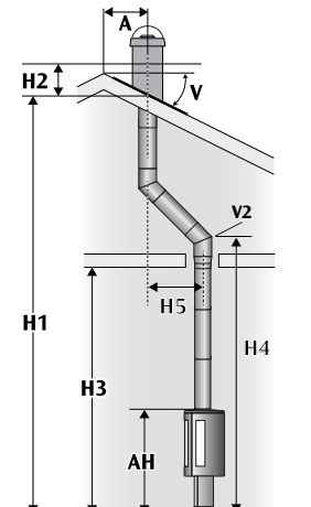
1TV - Toppansluten med halvisolerat startör och sidodragning.
