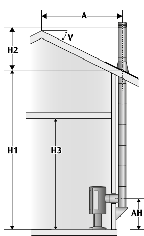
1BY - Bakansluten genom yttervägg
