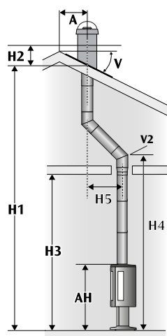
1TV - Toppansluten med halvisolerat start rör och sidodragning.
