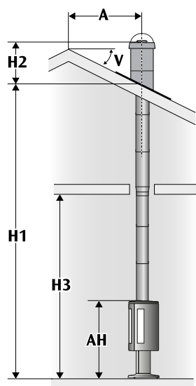
1T - Halvisolerat start rör med övergång dold i bjälklag.
