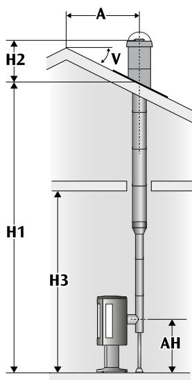
3B - Bakansluten direkt bakom eldstad. Oisolerat start rör.
