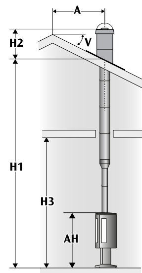
3T - Oisolerat start rör
