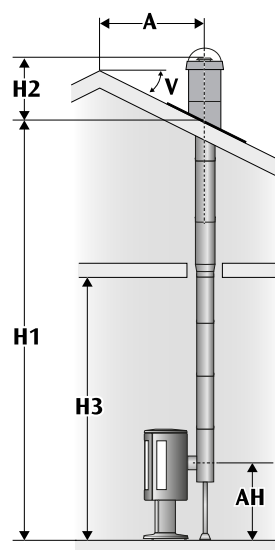
1B - Bakansluten direkt bakom eldstad. Halvisolerat start rör med övergång dold i bjälklag
