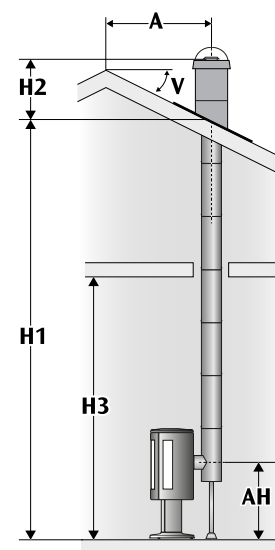
2B - Bakansluten direkt bakom eldstad. Helisolerad skorsten.
